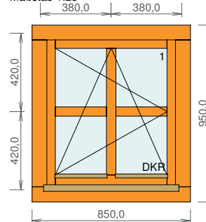
Pos. 3 4 Stück Maßstab 1:25
