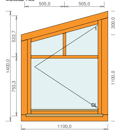
Pos. 6 1 Stück Maßstab 1:25
