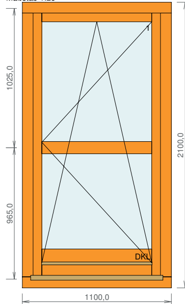
Pos. 5 1 Stück Maßstab 1:25
