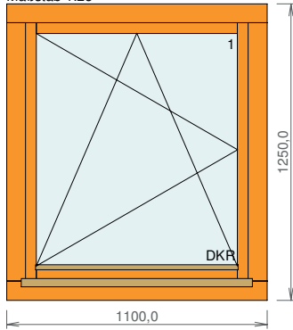
Pos. 1 2 Stück Maßstab 1:25
