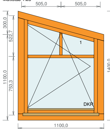
Pos. 5 1 Stück Maßstab 1:25
